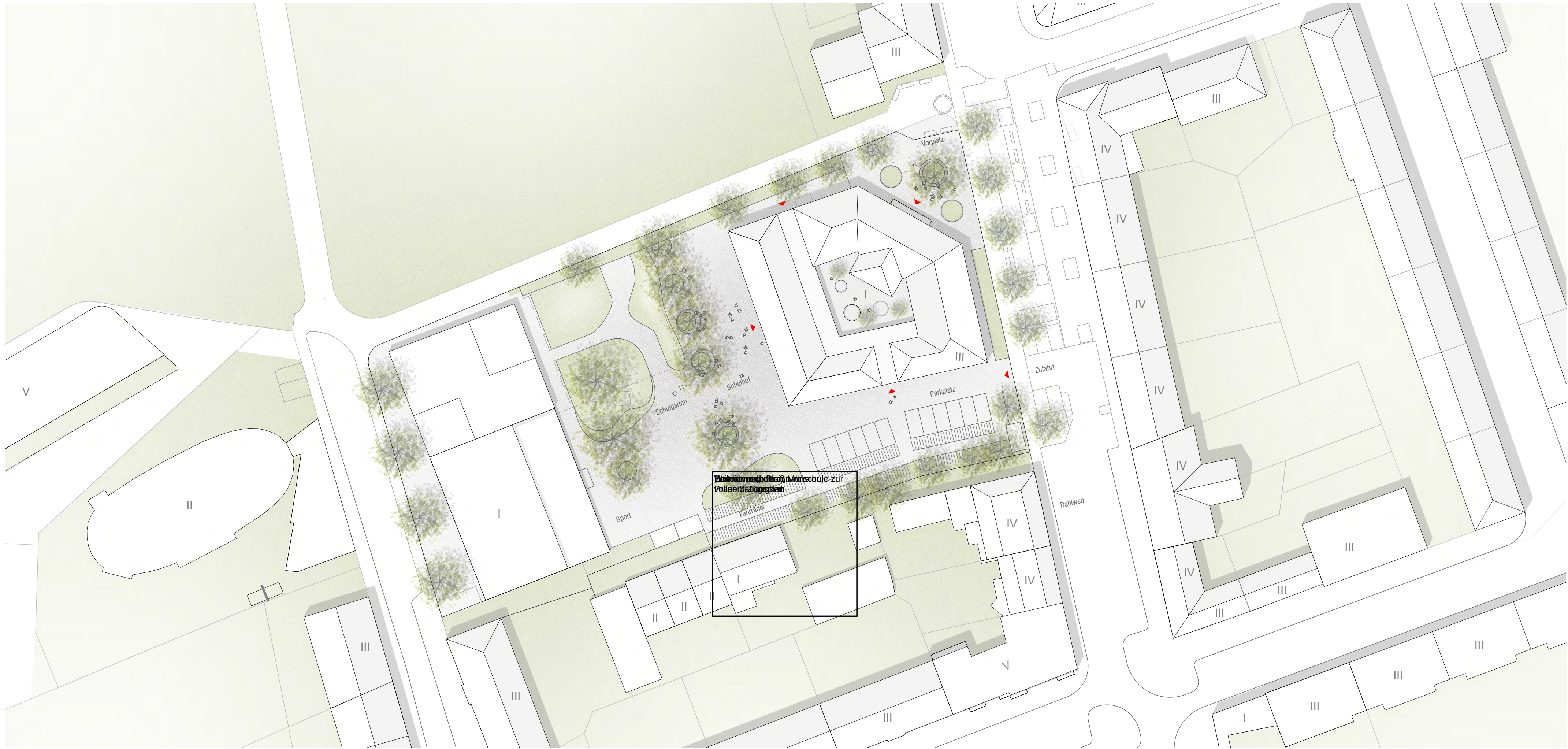
Lageplan 1:500
