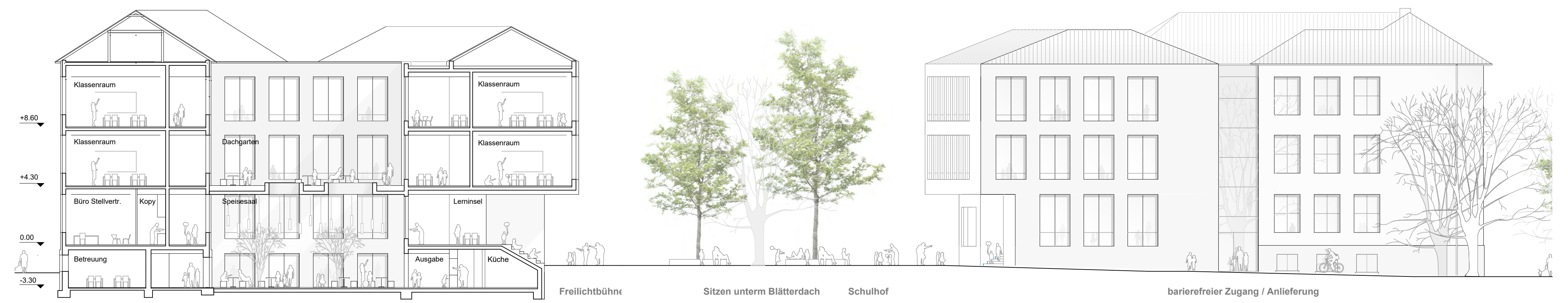
Schnitt A-A 1:200
