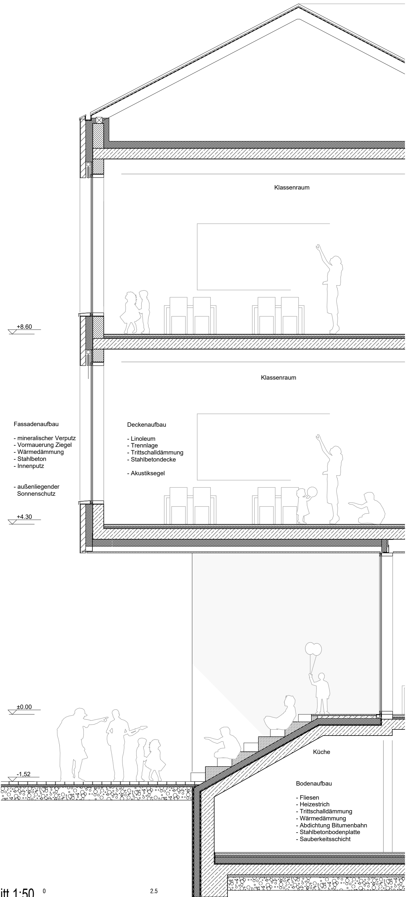
Fassadenschnitt 1:50
