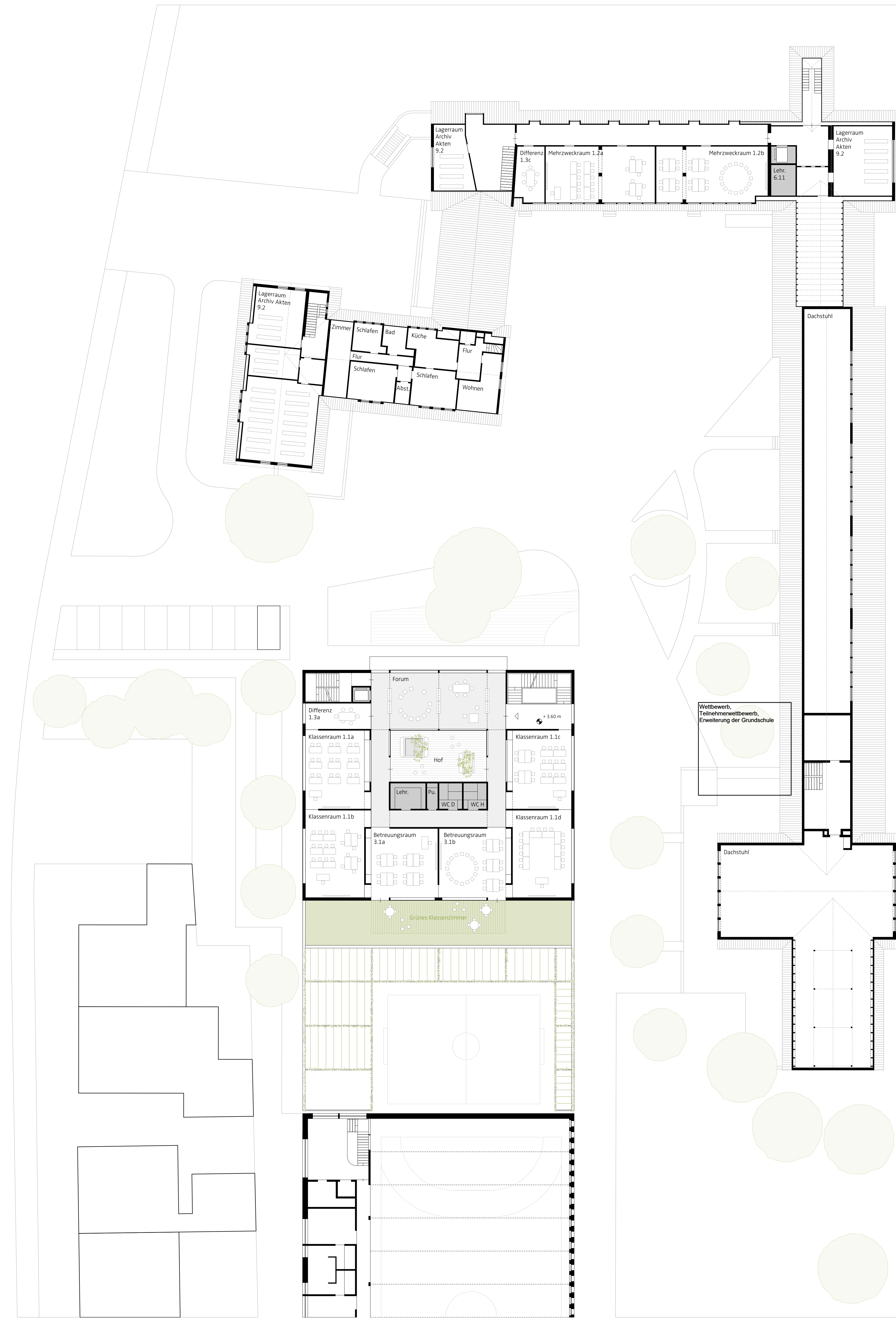
Grundriss OG I M 1:200
