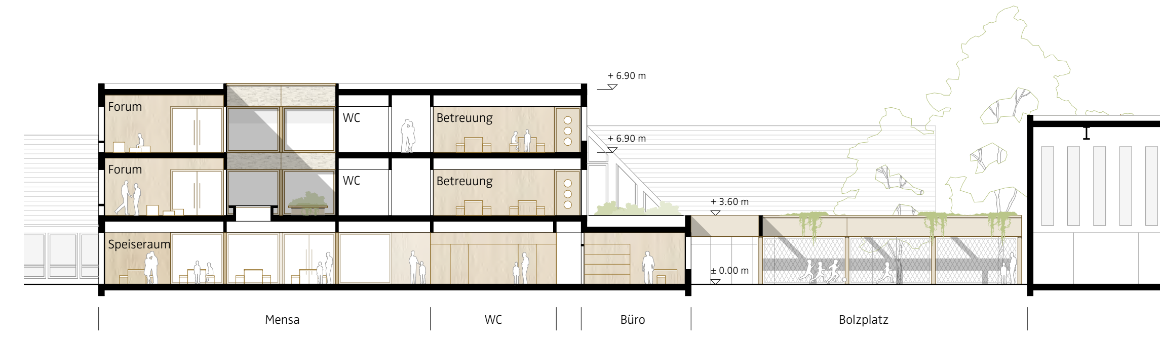
Schnitt B-B M 1:200
