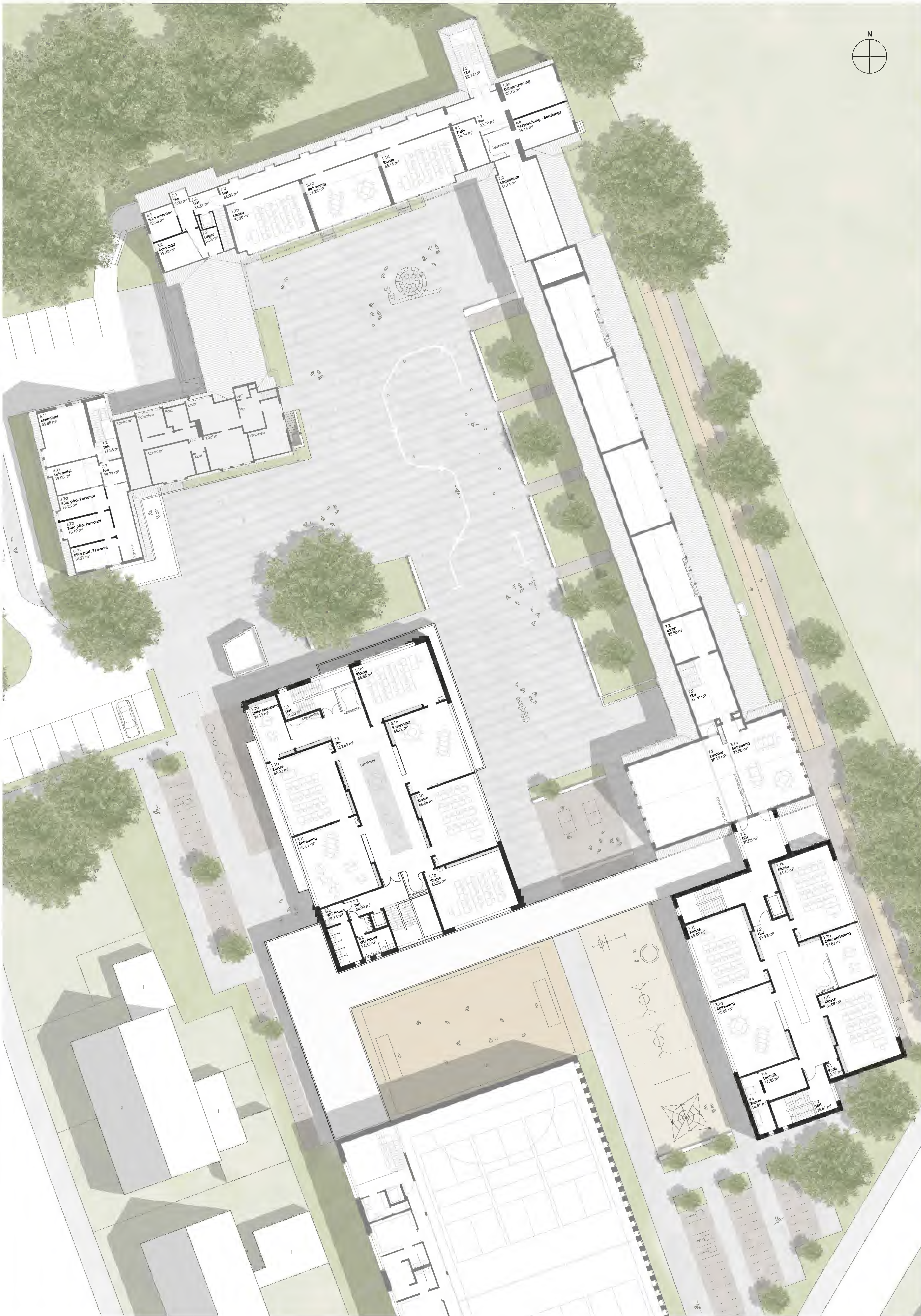
Grundriss Erdgeschoss M. 1:200
