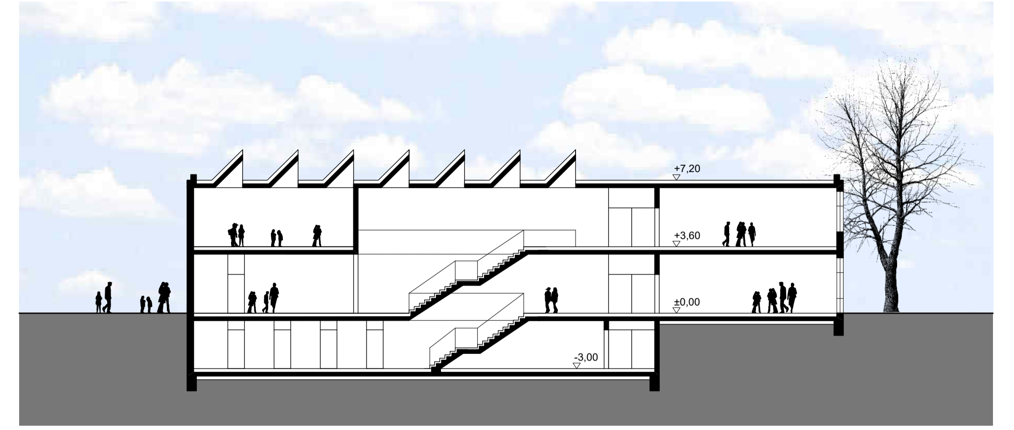
SCHNITT
