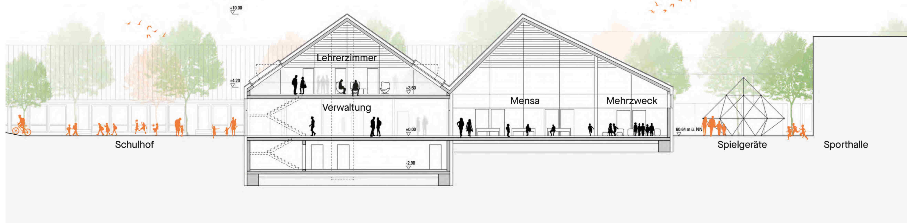
Schnitt BB M 1.200
