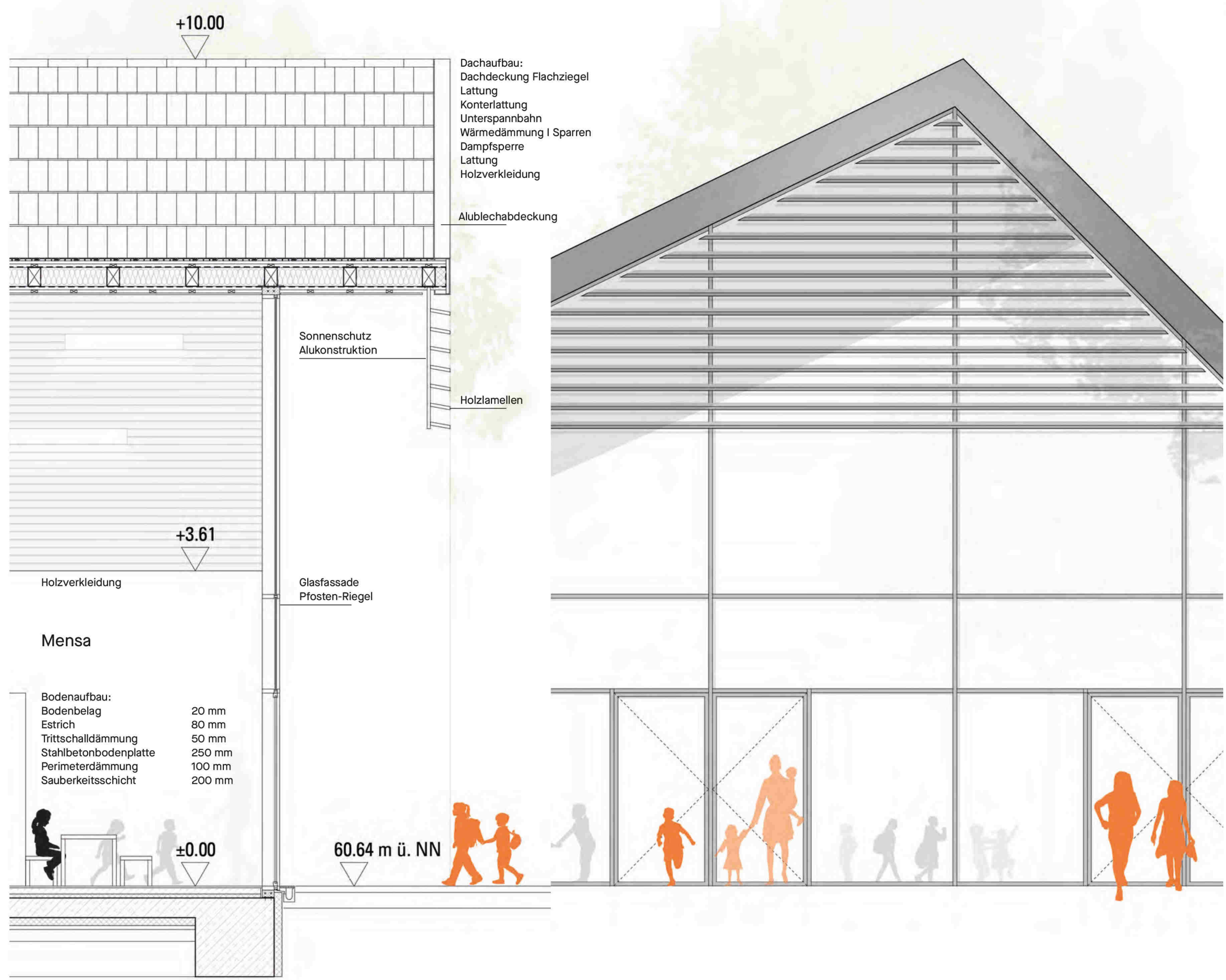
Fassadenschnitt M 1.50
