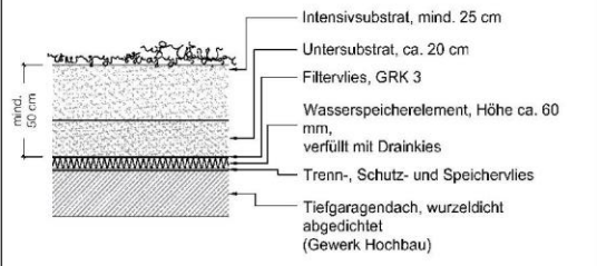
SCHEMASCHNITT GRÜNDACH AUF TIEFGARAGE, M 1:20
