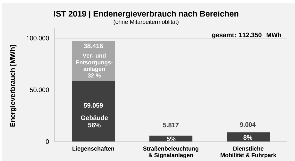
Abbildung 8: Ist 2019 | Endenergieverbrauch (ohne Mitarbeitermobilität) nach Bereichen der Stadtverwaltung Münster Quelle: IE Leipzig 2021
