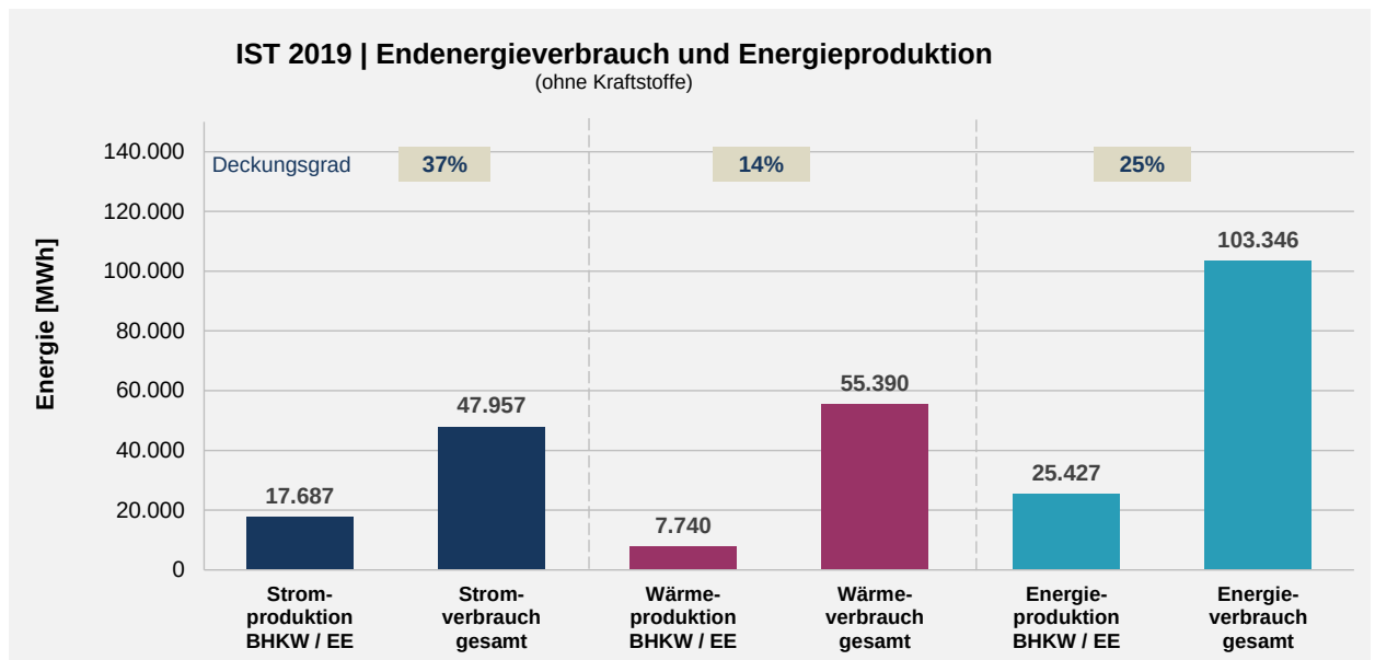
Abbildung 7: Ist 2019 | Endenergieverbrauch und Energieproduktion (ohne Kraftstoffe) der Stadtverwaltung Münster Quelle: IE Leipzig 2021
