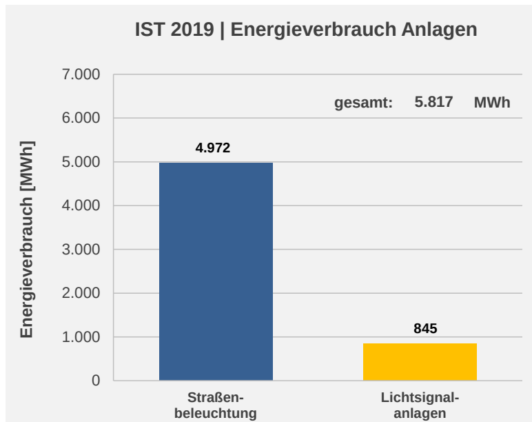
Abbildung 24: Ist 2019 | Energieverbrauch Straßenbeleuchtung und Lichtsignalanlagen der Stadtverwaltung Münster Quelle: IE Leipzig 2021
