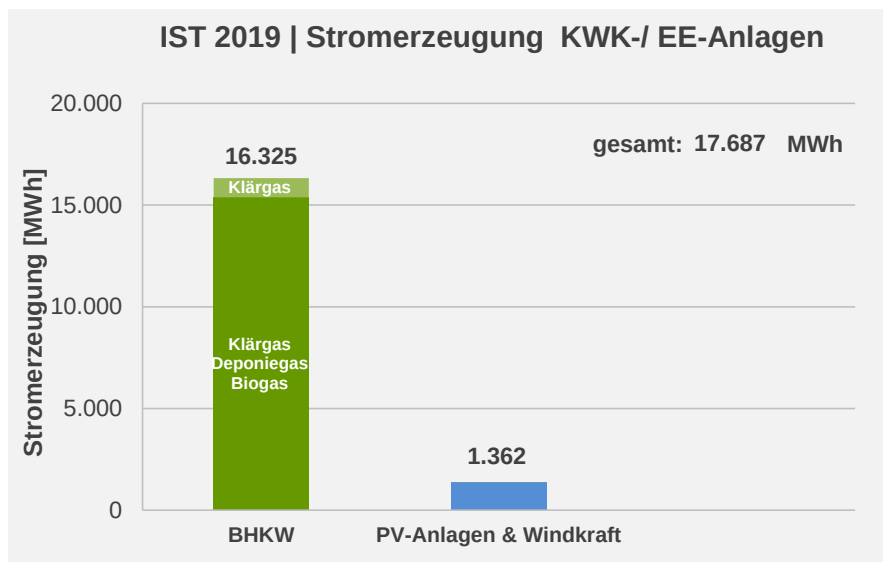
Abbildung 21: Ist 2019 | Stromerzeugung durch KWK / EE-Anlagen der Stadtverwaltung Münster
