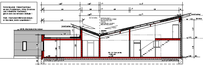
Schnitt Erweiterung
