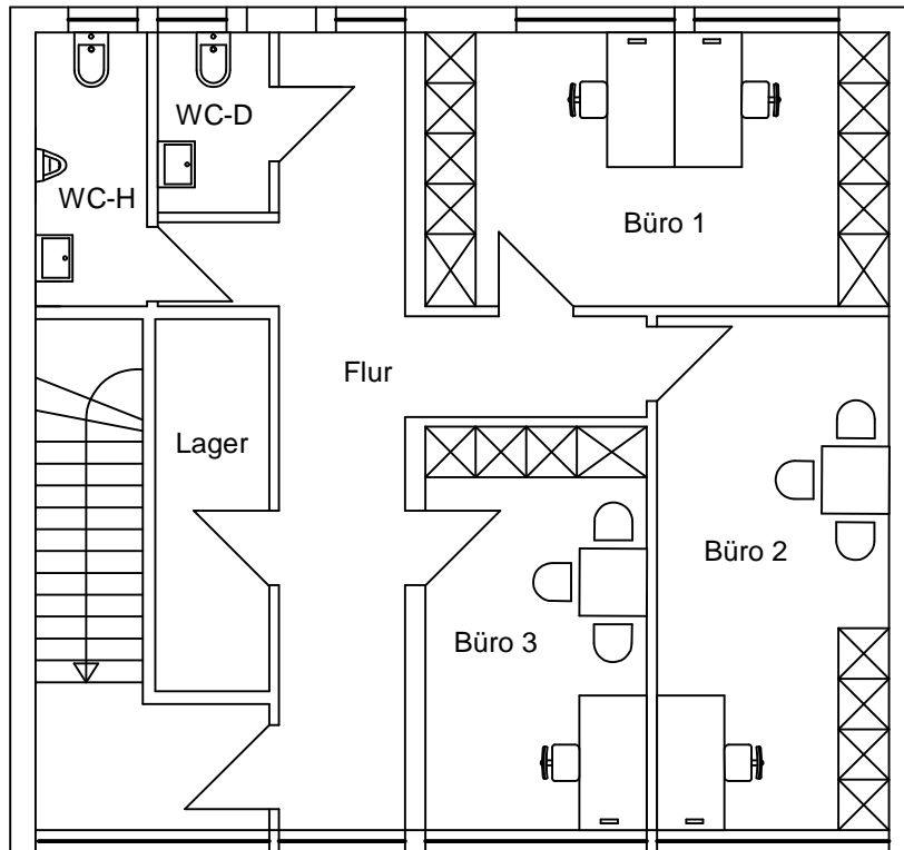
2. Obergeschoss
