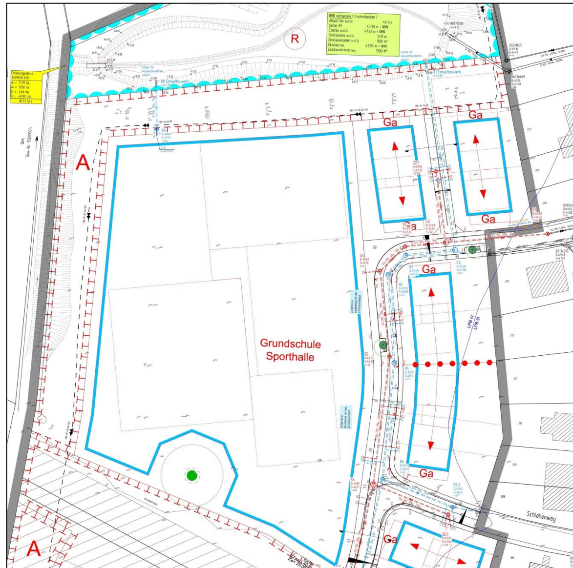
Kanalbau Lageplan Blatt Nr. 5
